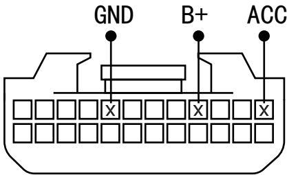
(24PIN连接器端子示意图)
